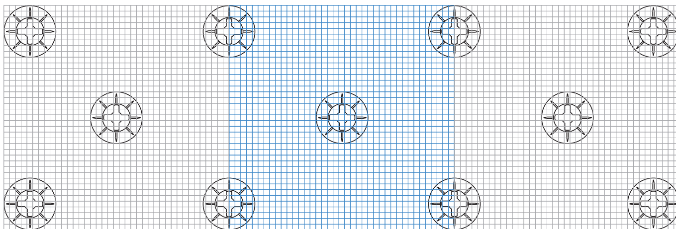
Eksempel på plassering av Flexi Level under gangbro (illustrert med 3 rister)
