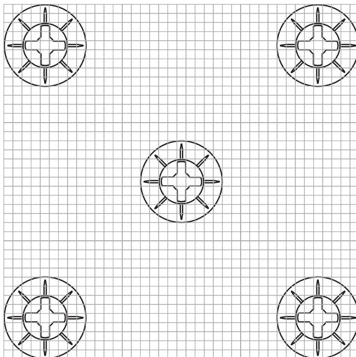
Eksempel på plassering av Flexi Level under en rist
